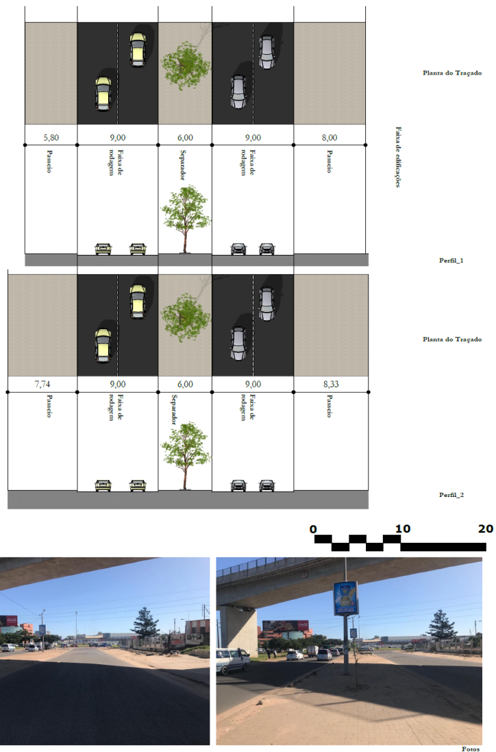
Figura 2. Plano de Traçado e perfil transversal da Av. 24 de Julho
